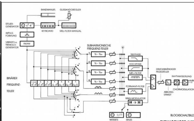
Prinzipschaltbild Subharchord II / III
